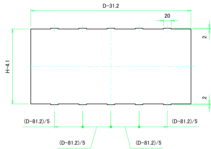
Dパネル1表面 / D Panel 1 Frontside
