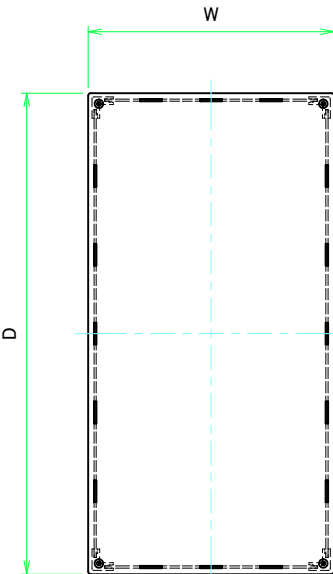
Wパネル1 / W Panel 1
